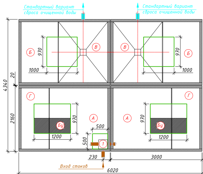
Схема станции
