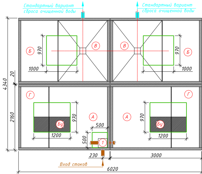
Схема станции
